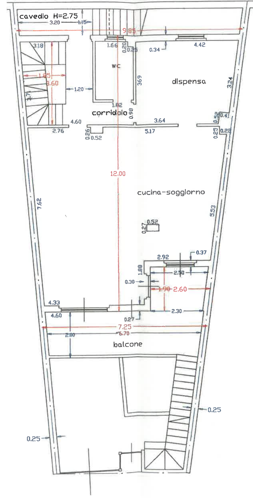
PIANO SEMINTERRATO h(grezzo) >> m. 2,70
